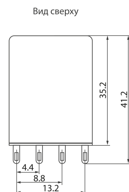
Реле промежуточное MY4
